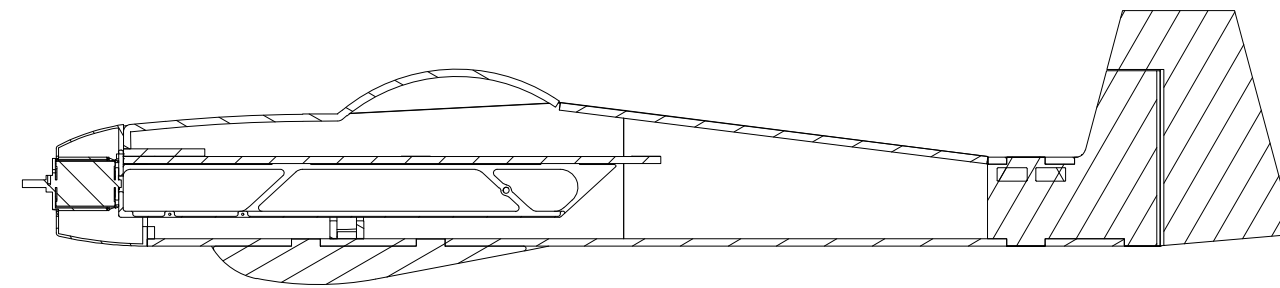
SECTION A-A SCALE: 1/5
