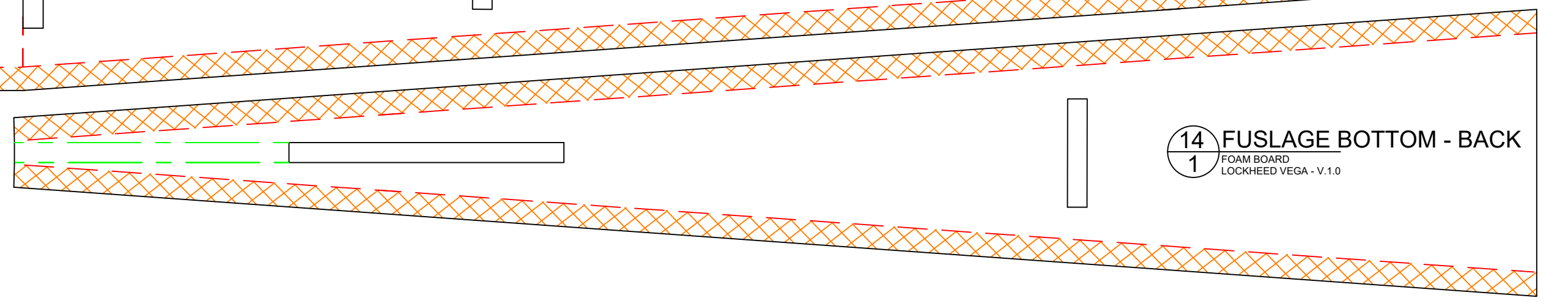
13 FUSLAGE TOP - BACK 1 FOAM BOARD LOCKHEED VEGA - V.1.0
